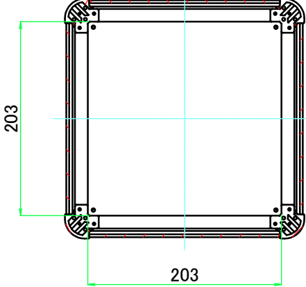
C-C ( 1 : 5.5 )
