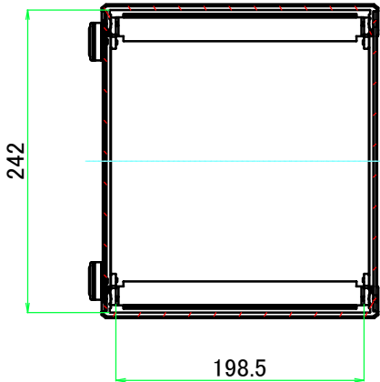
B-B ( 1 : 5.5 )
