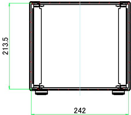
A-A ( 1 : 5.5 )
