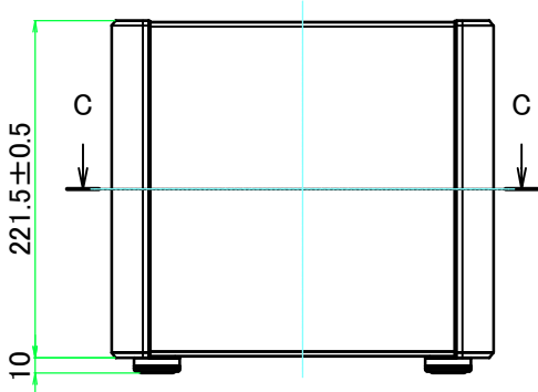
A-A ( 1 : 5.5 )
